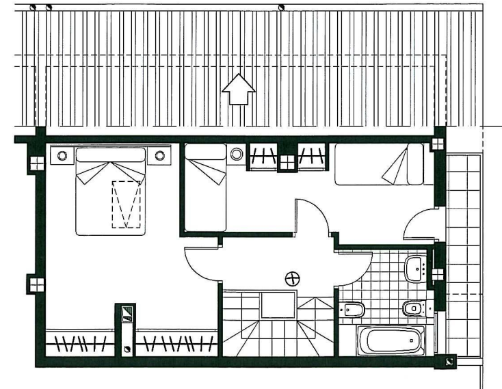
PLANTA ALTA DUPLEX
